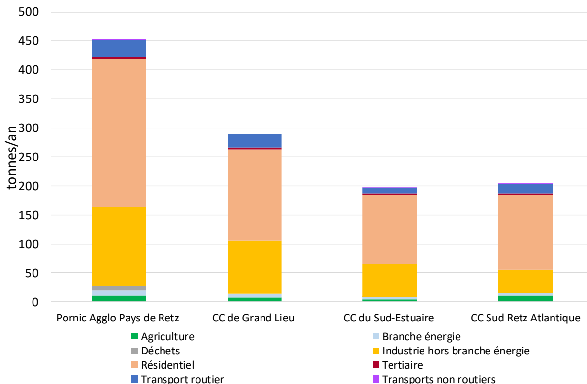
Figure 86 : Comparaison des répartitions des émissions de COVNM par secteur et par EPCI en 2016
