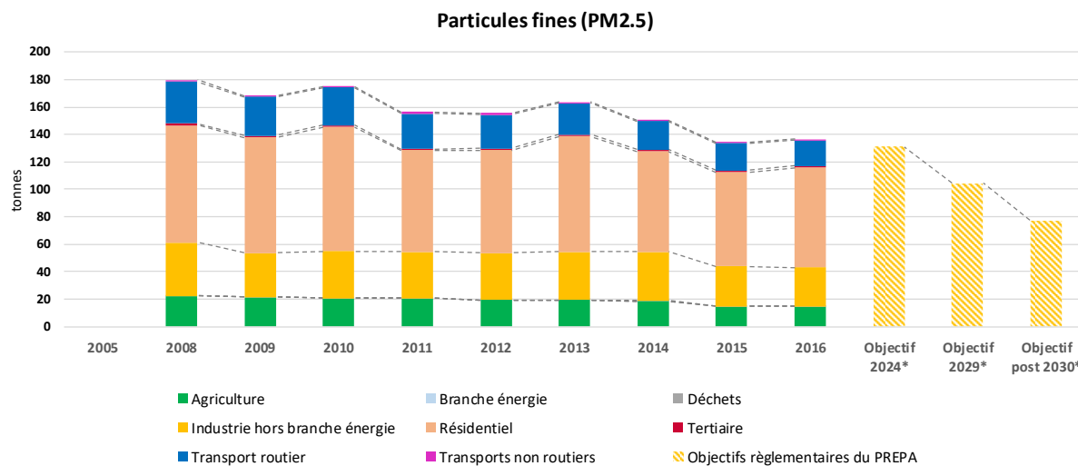
Figure 91 : Evolution des émissions de PM 2,5 sur la Communauté d'Agglomération Pornic Agglo Pays de Retz
