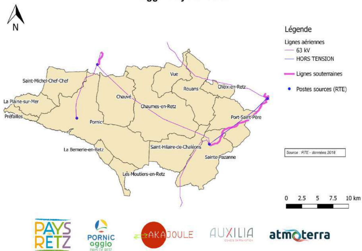
Figure 70 : Tracé du réseau de transport d'électricité
