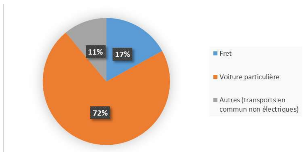
Figure 27 : Répartition des émissions énergétiques de GES du secteur routier par type de transport (à l'échelle de la CA Pornic Agglo Pays de Retz en 2016)
