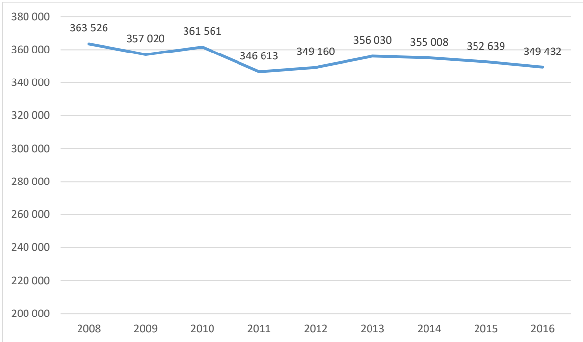
Figure 9 : Evolution des émissions territoriales de GES de Pornic Agglo Pays de Retz en t éq CO 2 sur la période 2008-2016
