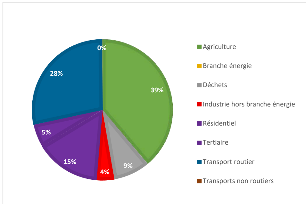
Figure 10 : Répartition des émissions territoriales de GES par secteurs à l'échelle de Pornic Agglo Pays de Retz (2016)
