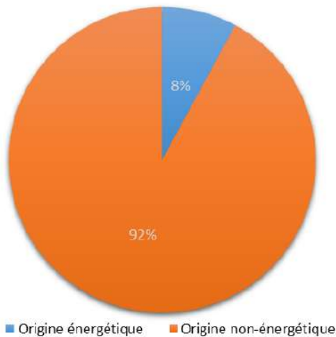
Figure 19 : Répartition des émissions de GES du secteur agricole par origine à l'échelle de la CA Pornic Agglo Pays de Retz en 2016
