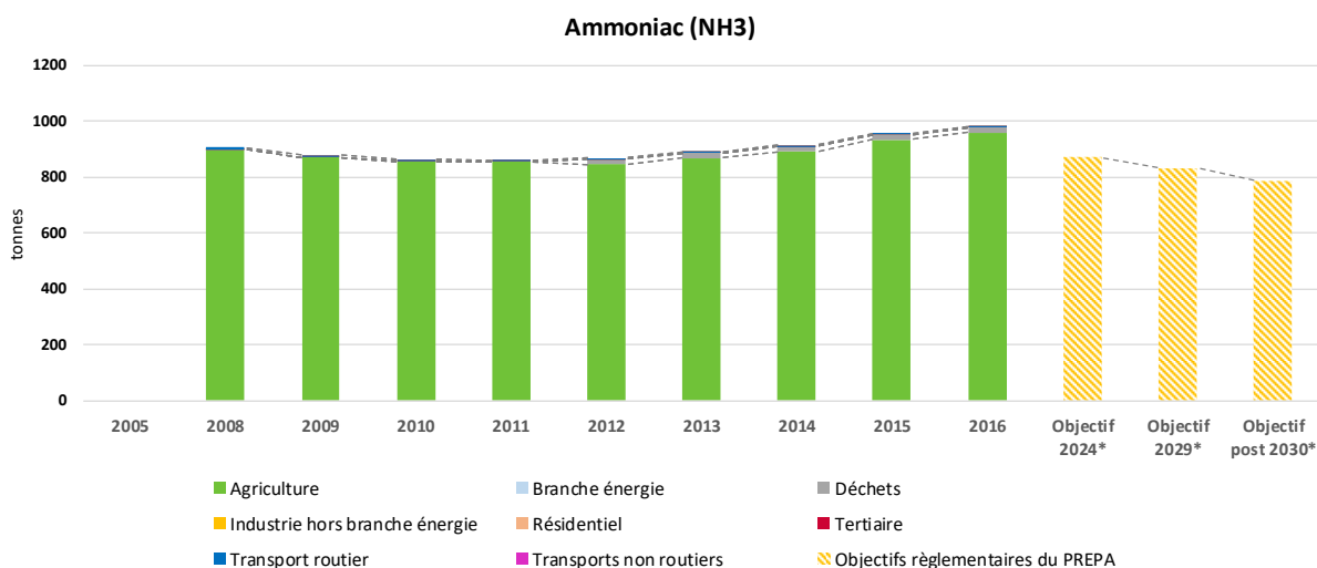
Figure 92 : Evolution des émissions de NH 3 sur la Communauté d'Agglomération Pornic Agglo Pays de Retz Source : BASEMIS / AIR PAYS DE LA LOIRE
