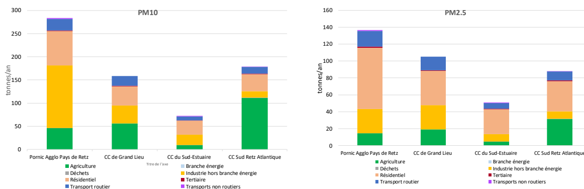
Figure 84 : Comparaison des répartitions des émissions de particules fines par secteur et par EPCI en 2016
