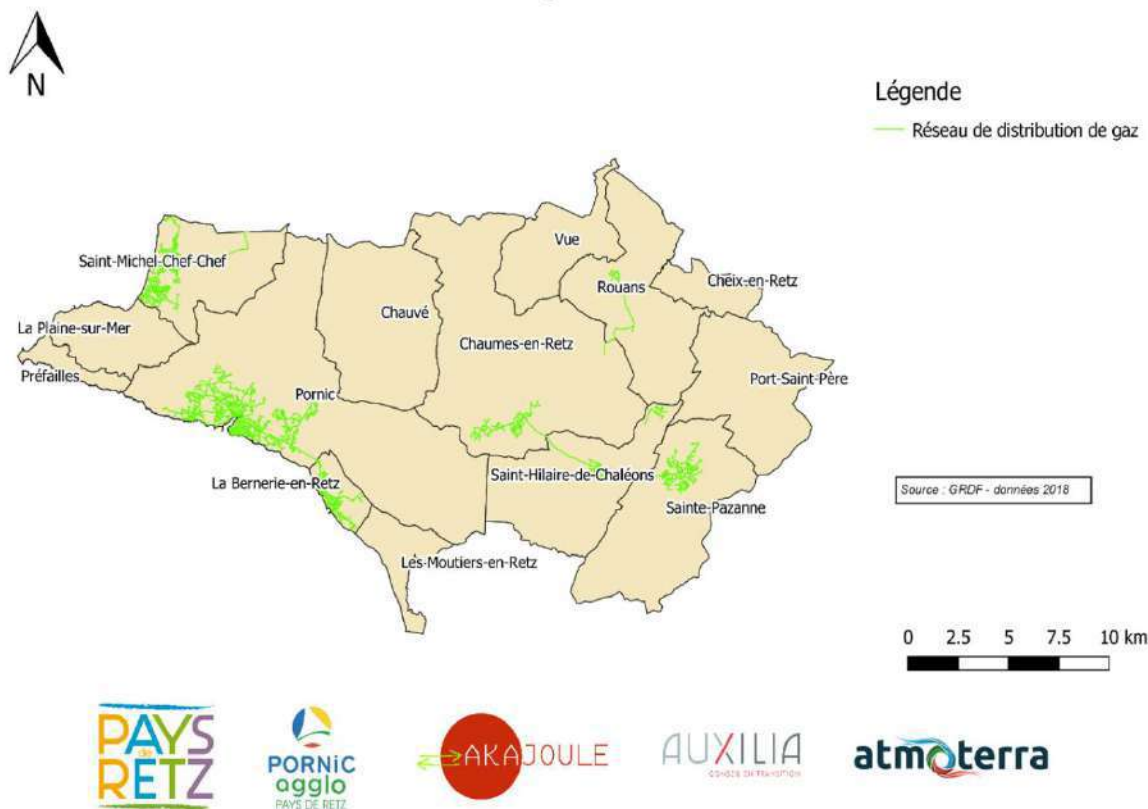
Figure 73 : Tracé du réseau de distribution de gaz Source : GRDF
