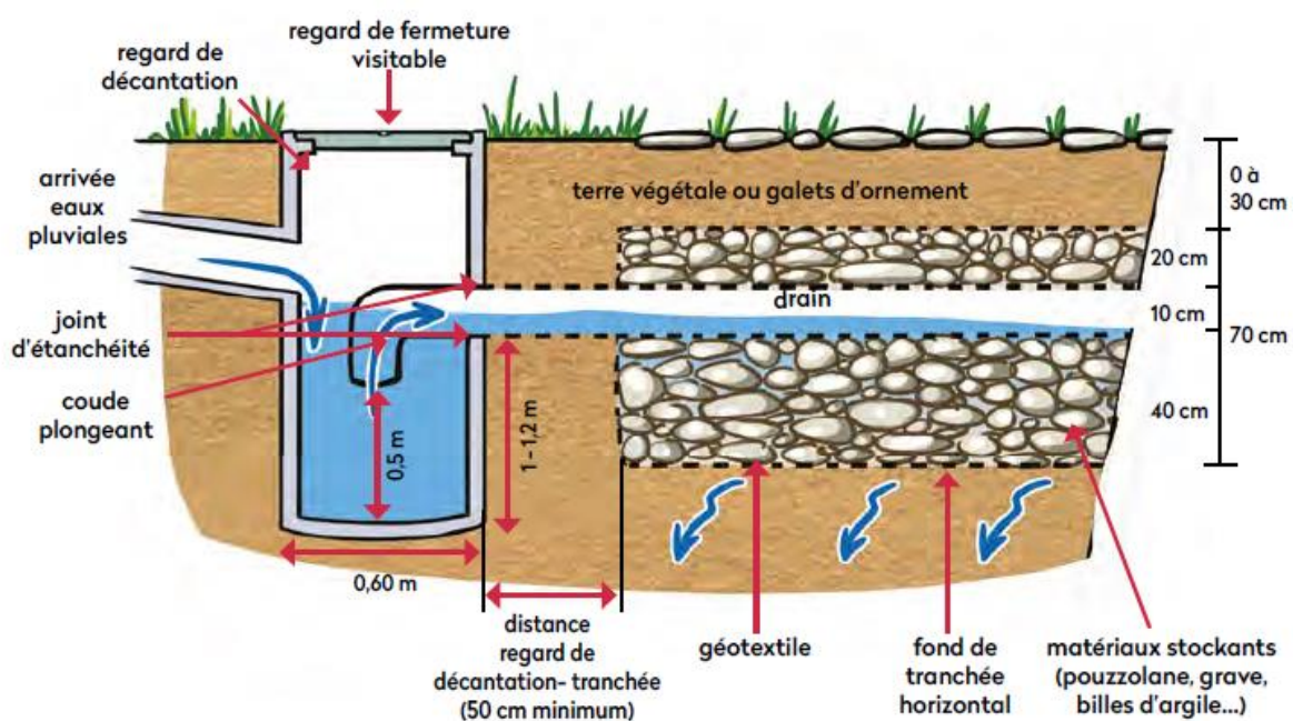
Figure 2 : Exemples de coupes de tranchées
