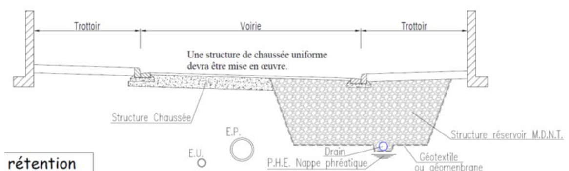
Figure 8 : Coupe d'une chaussée à structure réservoir
